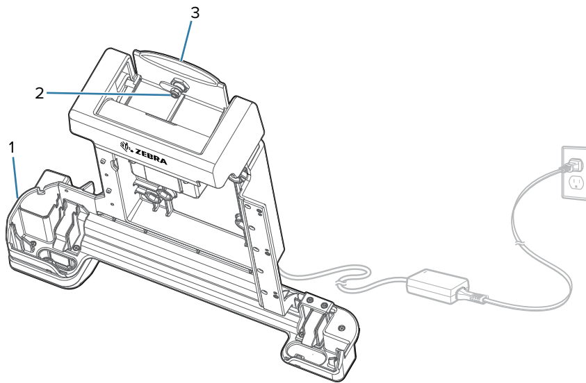
Figura 3 Configuración de la base de solo alimentación
