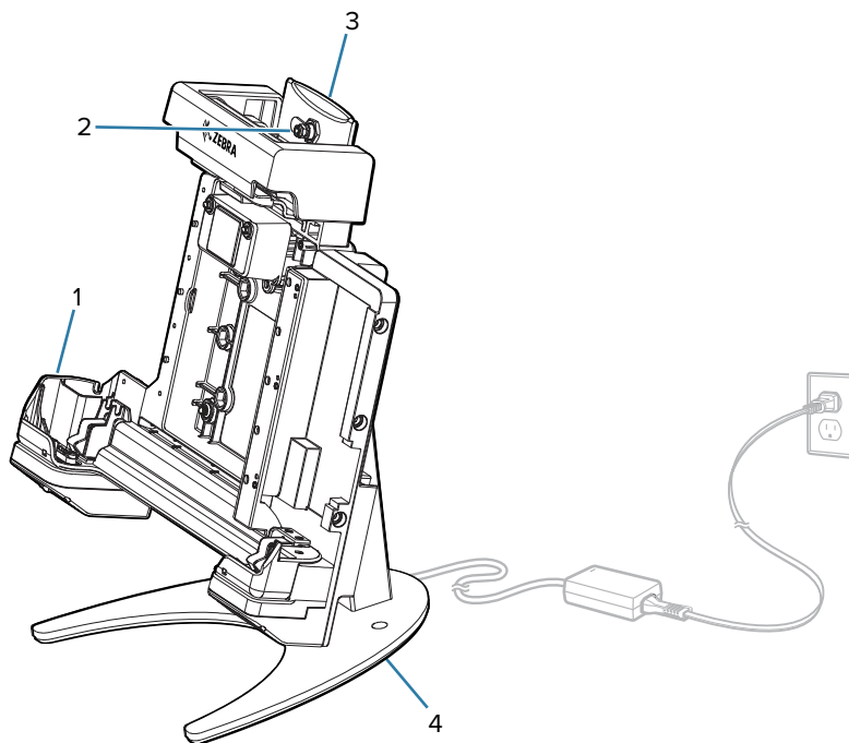
Figura 5 Instalación de la base para oficina
