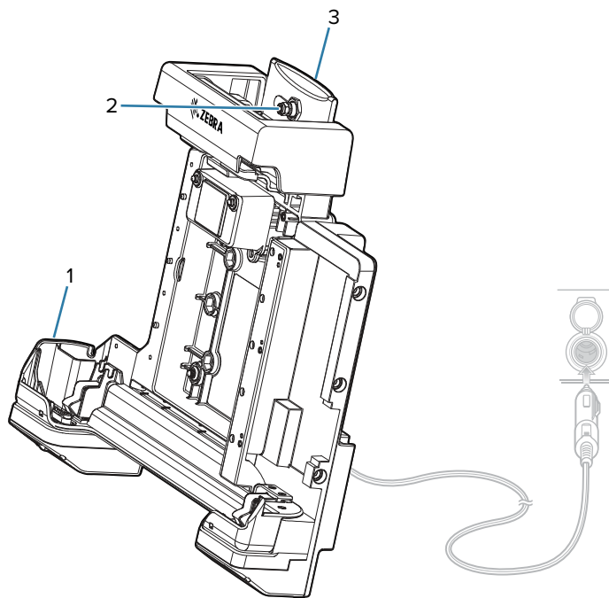
Figura 4 Configuración de la base para vehículo
